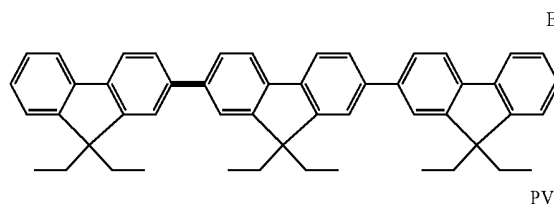
PVK
